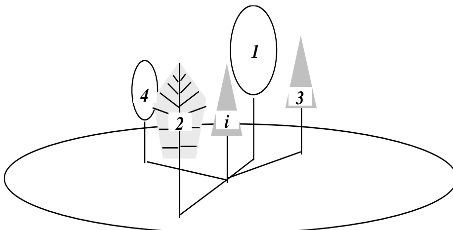
Figura 1. Representación gráfica del grupo estructural de cinco árboles
